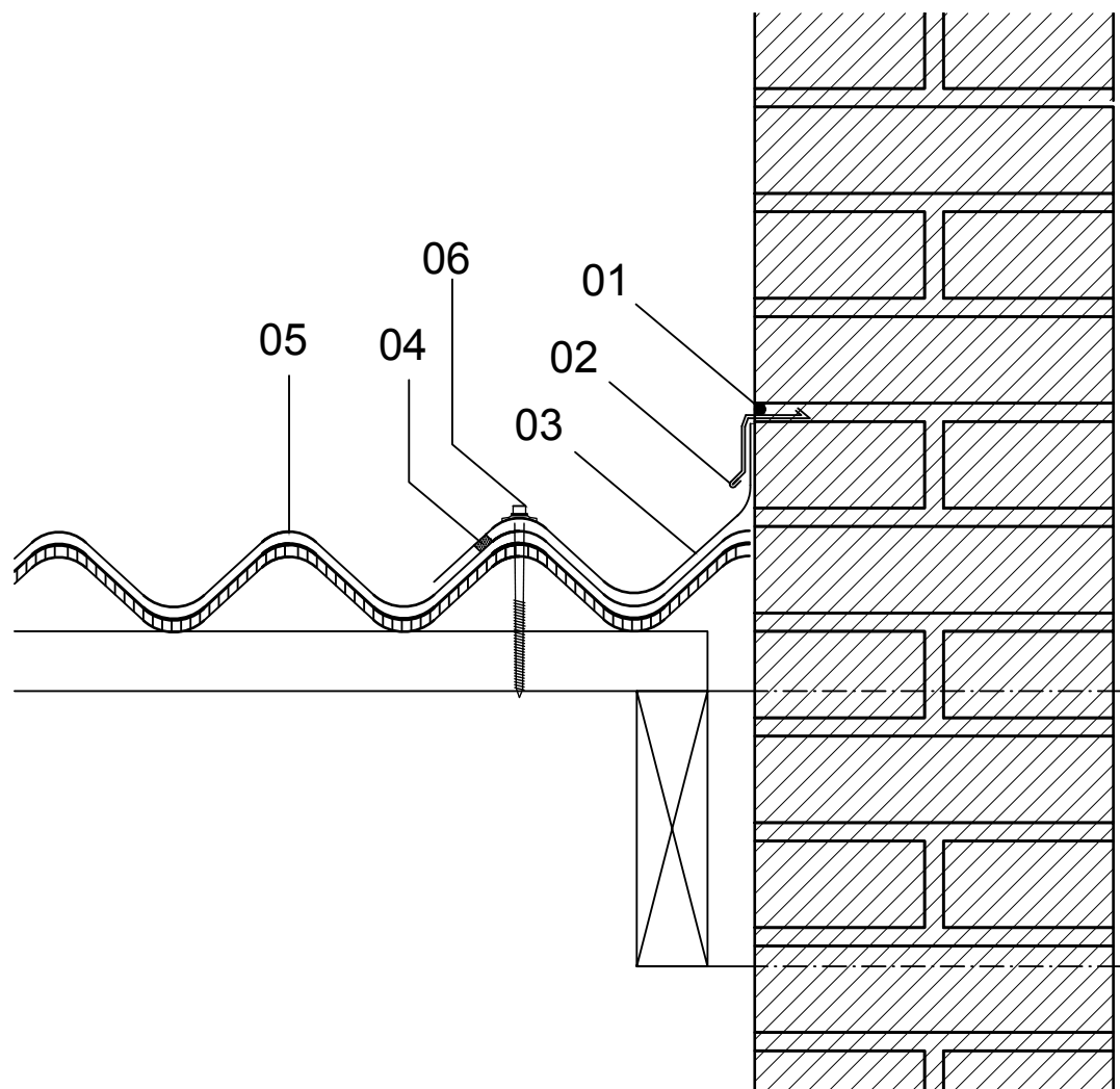
Lodrätt snitt - anslutning skorsten
